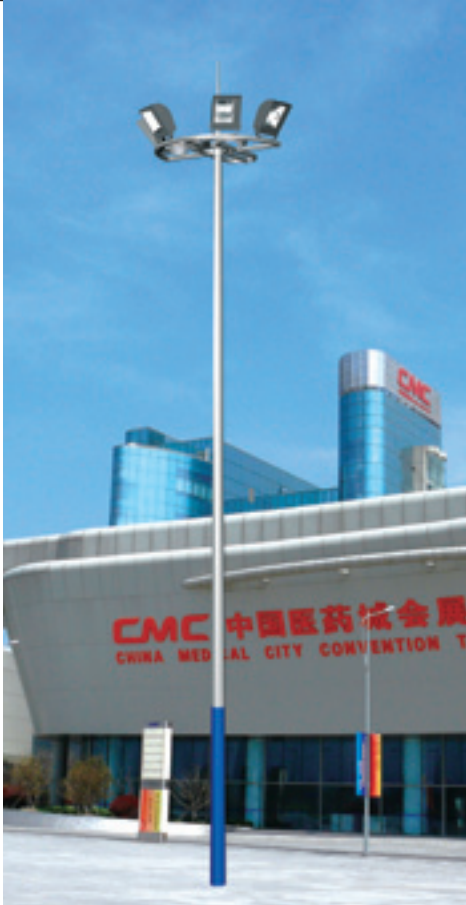
型号: LDZG-18201 型 高度: 13-16m 光源: 钠灯 / 节能灯 / 金卤灯
